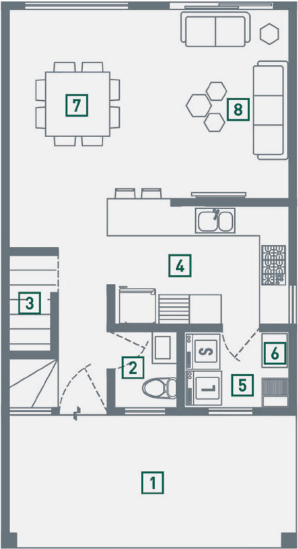
PLANTA BAJA
